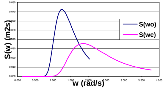
Figura6: Para un análisis realizado con un estado de mar 3, 8 nudos y 75% de su desplazamiento.
