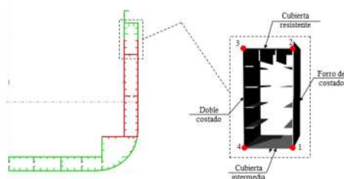
Figura 2. Definición de la cuaderna maestra y el cajón de torsión.
