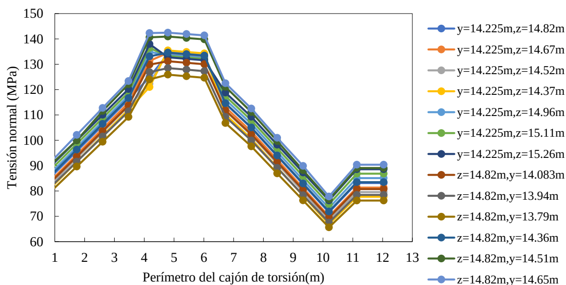
Figura 7. Evolución de las tensiones normales del buque viga a lo largo del perímetro del cajón de torsión.
