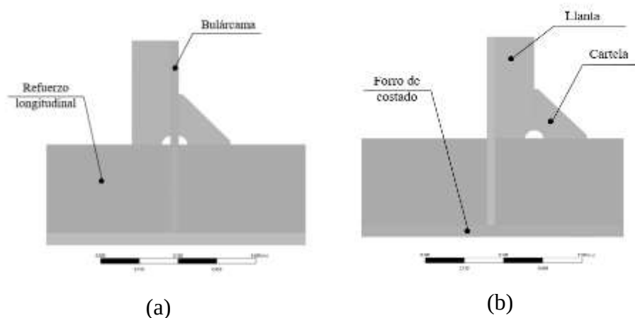
Figura 4. (a) Det3 y (b) Det6
