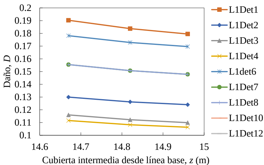
Figura 5. Evolución del daño por fatiga para el longitudinal n° 1 (L1) bajo la modificación de los valores de punta de la cubierta intermedia y diferentes detalles estructurales.
