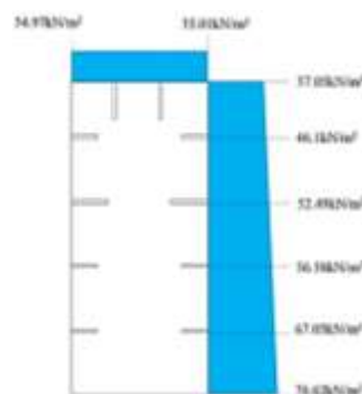
Figura 3. Valores máximos de presión (hidrostática + dinámica).
