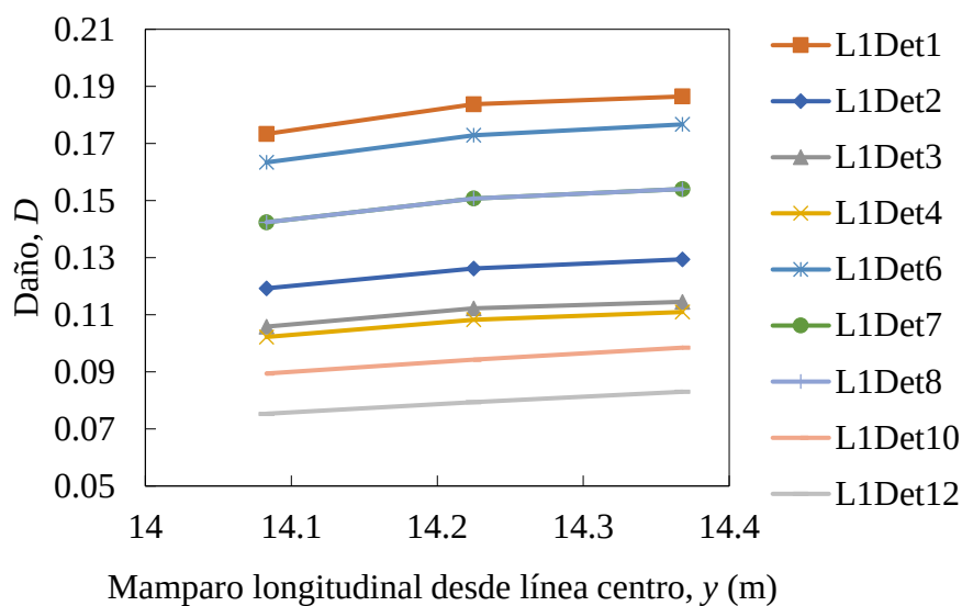
Figura 6. Evolución del daño por fatiga para el longitudinal nº 1 (L1) bajo la modificación de los valores del mamparo longitudinal y los diferentes detalles estructurales.
