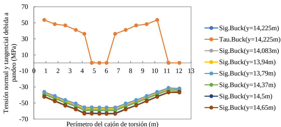
Figura 9. Evolución de la tensión crítica de pandeo, normal (Sig. Buck) y tangencial (Tau. Buck), a lo largo del perímetro del cajón de torsión para los diferentes valores de la manga.
