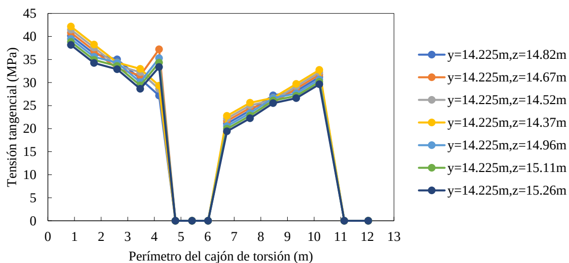
Figura 8. Evolución de las tensiones tangenciales del buque viga a lo largo del perímetro del cajón de torsión.
